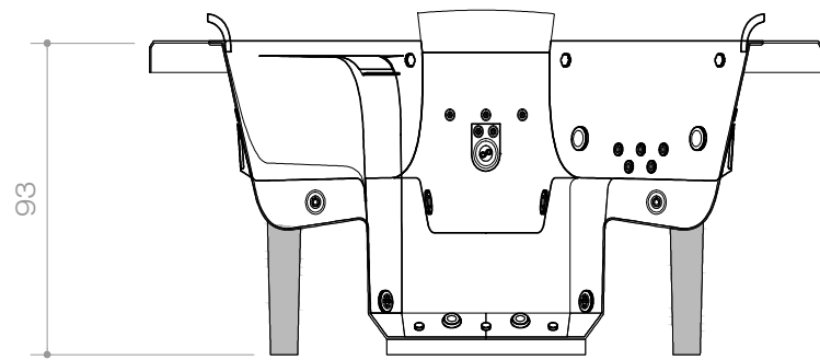
Corte AA'
