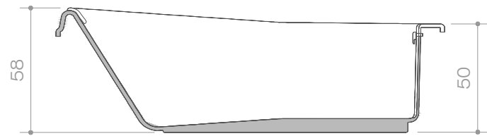
Corte AA'
