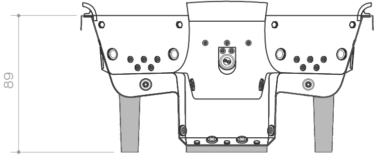
Corte AA'
