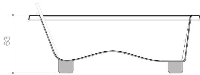
Corte AA'
