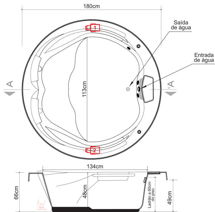
Corte AA'
